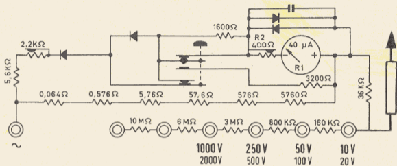
Circuito semplificato Voltmetro in C.A.
