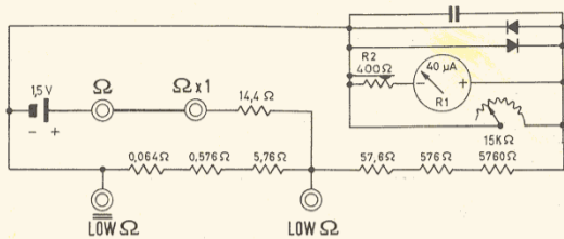
Schema semplificato Ohmetro per bassi valori.
