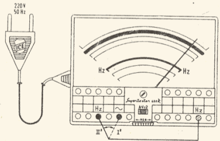
Schema come impiegare il Supertester 680 R per misure di frequenza
