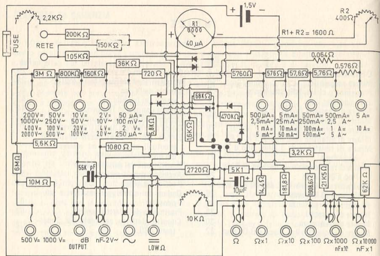
SCHEMA ELETTRICO DEL SUPERTESTER 680/R I.C.E. - 6ª serie
