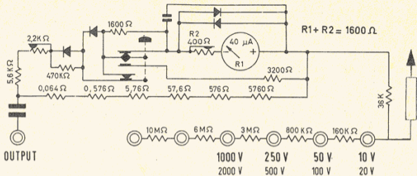
Schema semplificato misuratore d'uscita (Output)
