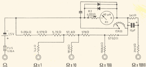
Circuito semplificato Ohmetro in C.C.
