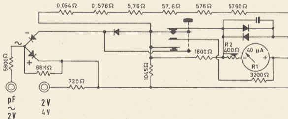
Circuito semplificato Voltmetro 2 e 4 Volts in C.A.
