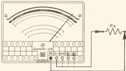
Schema come misurare le resistenze col supertester 680 R
