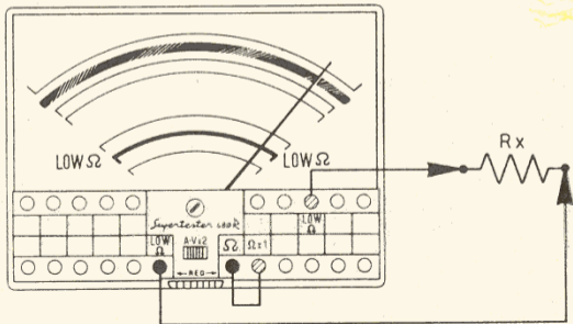
Schema semplificato Ohmetro per bassi valori.
