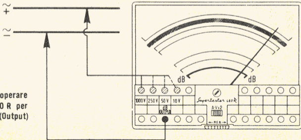
Schema semplificato misuratore d'uscita (Output)
