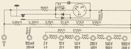
Schema semplificato del Voltmetro in C.C.
