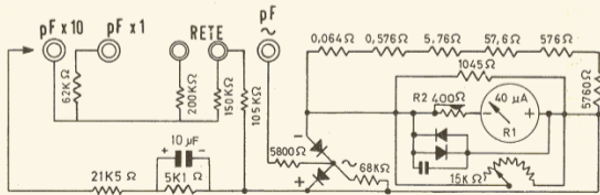
Schema semplificato misuratore di capacità
