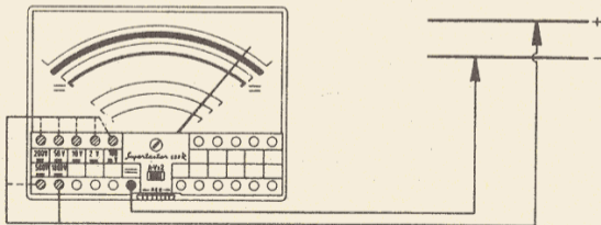
Schema come va inserito il SUPERTESTER 680 R nel circuito Voltmetrico in C.C.
