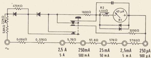
Circuito semplificato amperometro - in corrente alternata.
