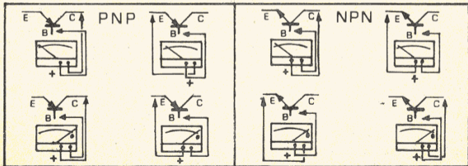
Posizione indice per la prova da transistors.
